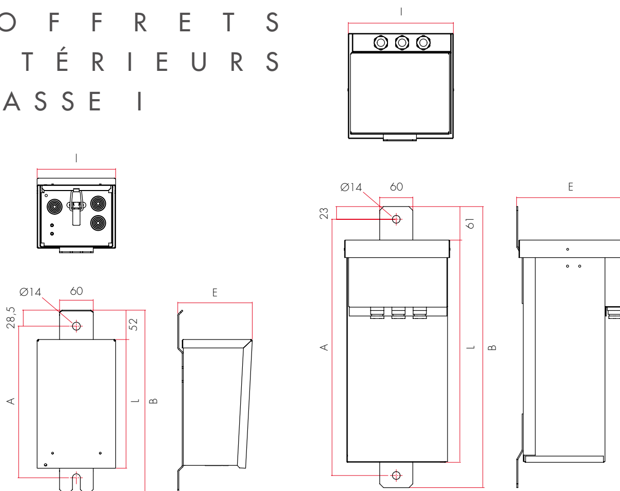
Coffret VB1 inox
