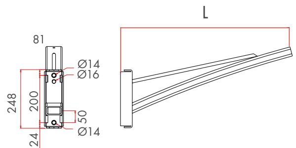
• KÉALIT MURAL 750 AND 1200
