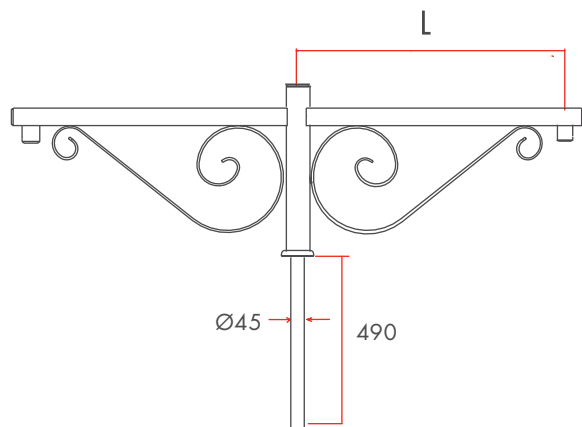
• VÉRONÉ DOUBLE LIGHTS
