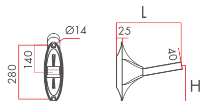
• KEALIT MURALE ET FEU DÉCALÉ 300
