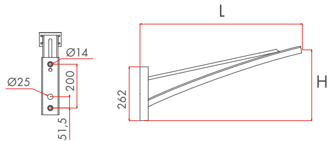
• KEALIT MURALE 750 ET 1200
