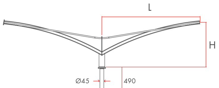
• KÉALIT DOUBLE FEU
