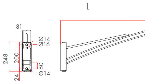
• KÉALIT MURALE 750 ET 1200
