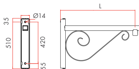
VÉRONE MURALE ET FEU DÉCALÉ SUSPENDUE 500 MM (ENTRAXE 310 MM), 750 ET 1000 MM (ENTRAXE 420 MM)
