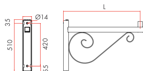
VÉRONE MURALE ET FEU DÉCALÉ PORTÉE 500 MM (ENTRAXE 310 MM), 750 ET 1000 MM (EN- TRAXE 420 MM)
